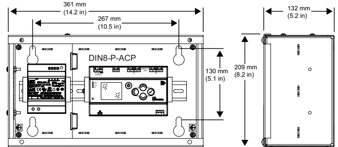
DIN8-P-ACP Front
